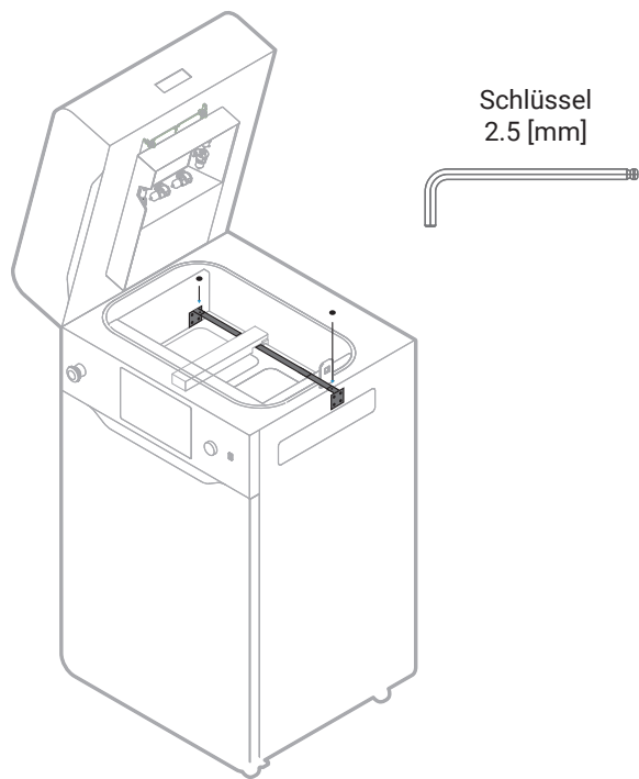
Abb. 5 Schrauben des Strips.
